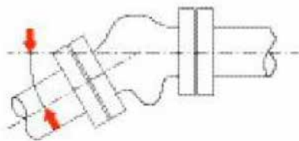
Mouvement angulaire
